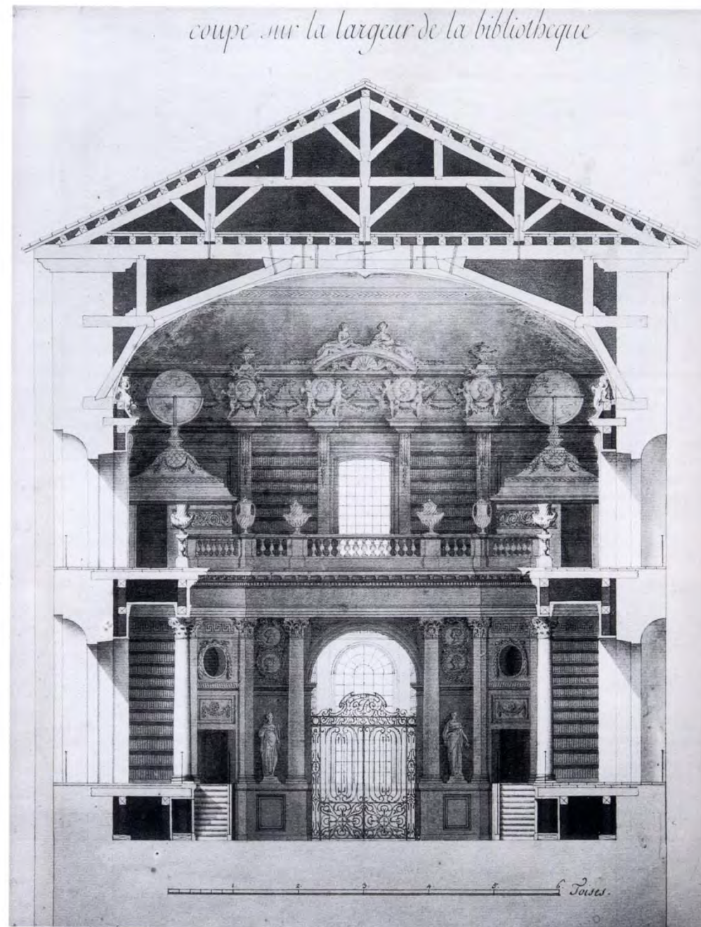
Fig. 93 – Spaccato di gran sala da biblioteca. Ubicazione ignota.
